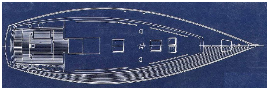
afb. 2 V42C bovenaanzicht dekindeling
