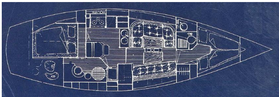
afb. 1 V42C bovenaanzicht binnenindeling
