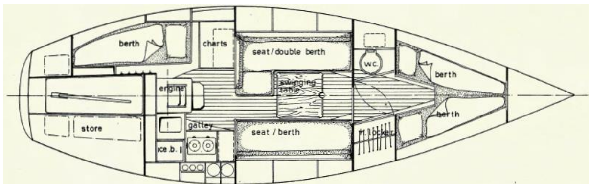
afb. 1 Binnen-indeling 1976-1992 bovenaanzicht
