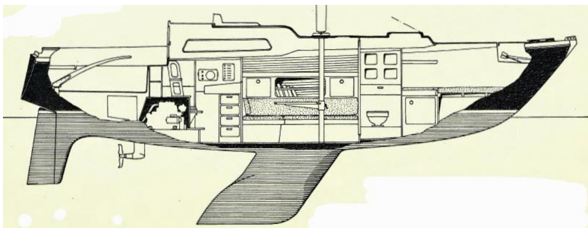
afb. 2 Binnen-indeling 1976-1992 zijaanzicht
