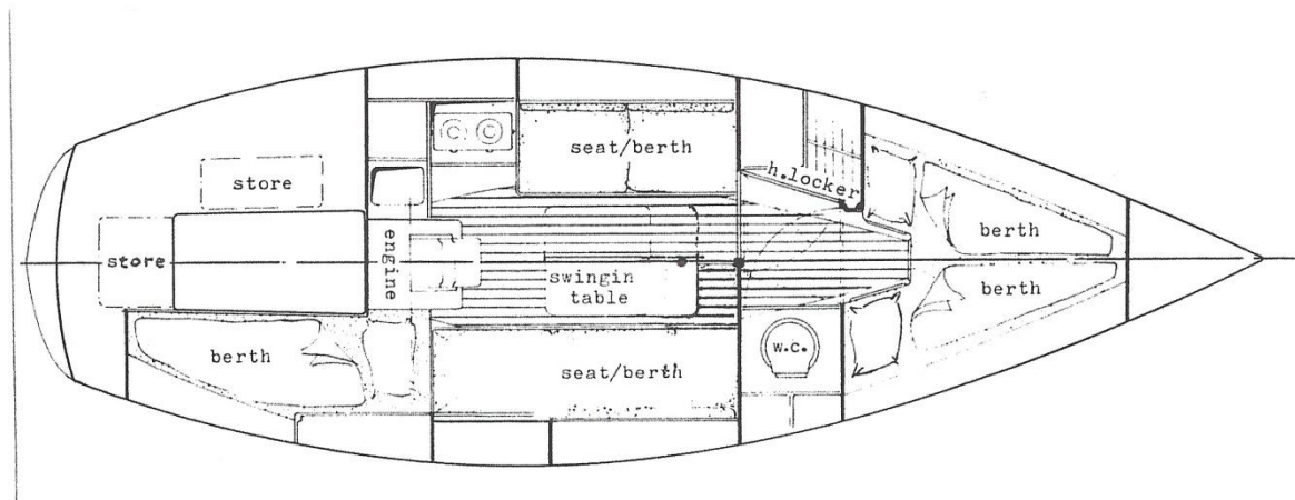
afb. 2 Bovenaanzicht binnenindeling met langsbank
