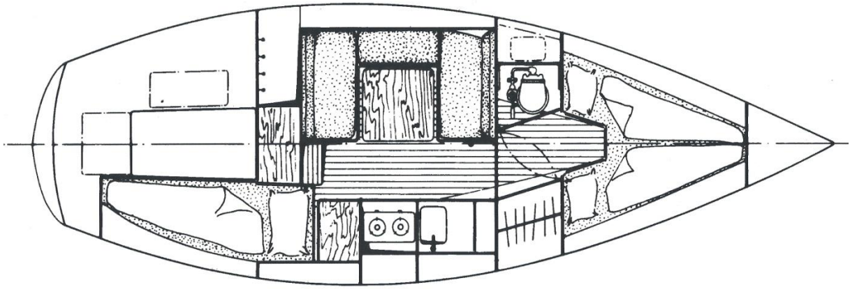
afb. 1 Bovenaanzicht binnenindeling met U-bank
