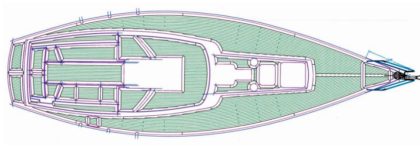
afb. 2 Bovenaanzicht dekindeling
