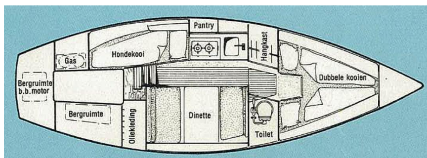
afb. 1 Bovenaanzicht binnenindeling V26
